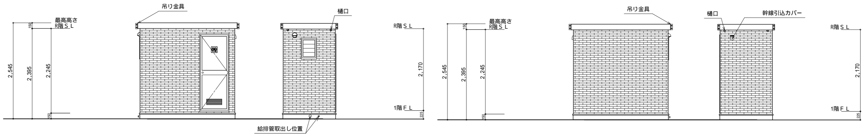
A側 立面図 S:1/60
